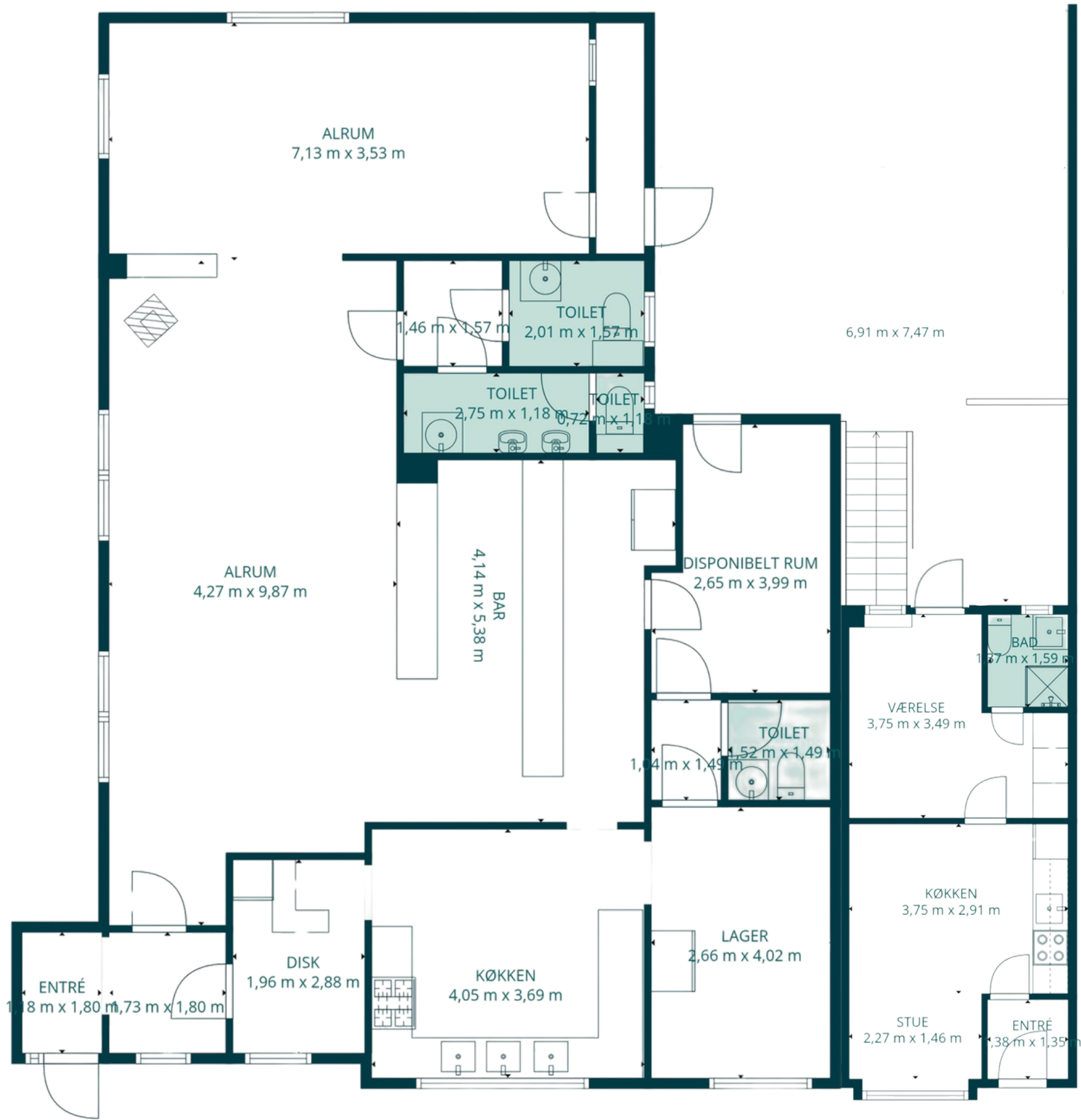
STUEPLAN
