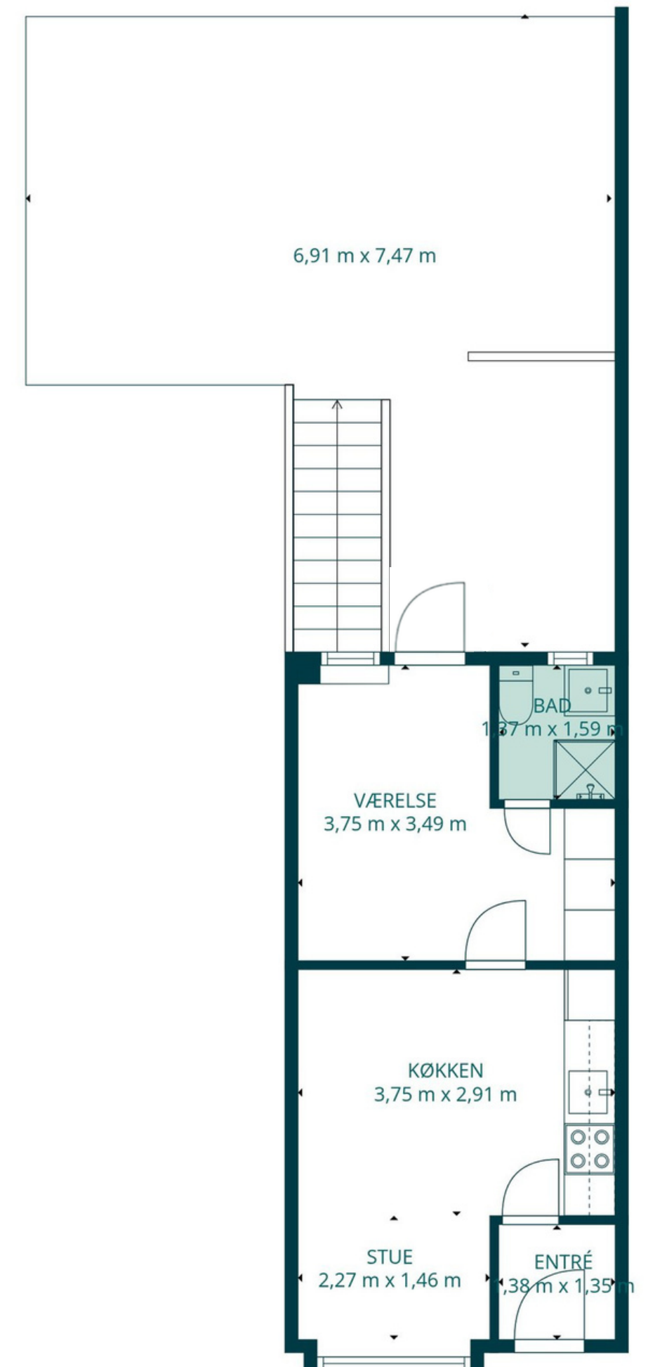
STUEPLAN
